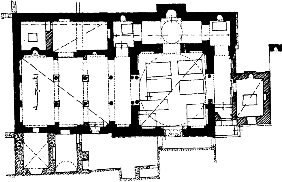
ضريح يحيى الشيبى القديم
